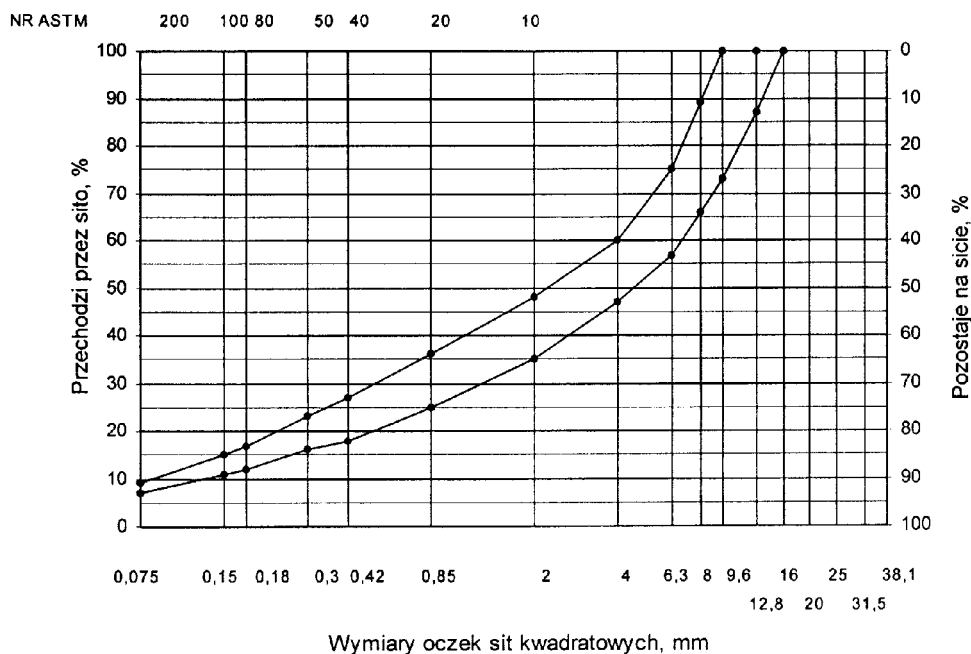
Rys. 4. Krzywe graniczne uziarnienia mieszanki mineralnej BA od 0 do 12,8 mm do warstwy ściernalnej nawierzchni drogi o obciążeniu ruchem od KR3 do KR6
