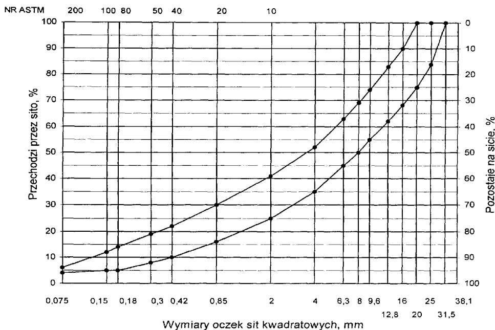
Rys. 5. Krzywe graniczne uziarnienia mieszanki
